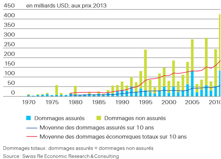
Figure 17. Évolution des dommages assurés et non assurés causés par les catastrophes naturelles dans le monde, depuis 1970
